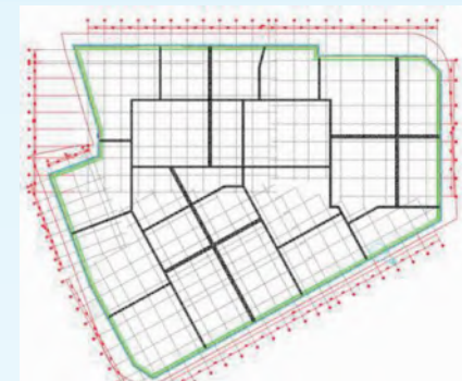
设计最终调整后的底板后浇带划分
