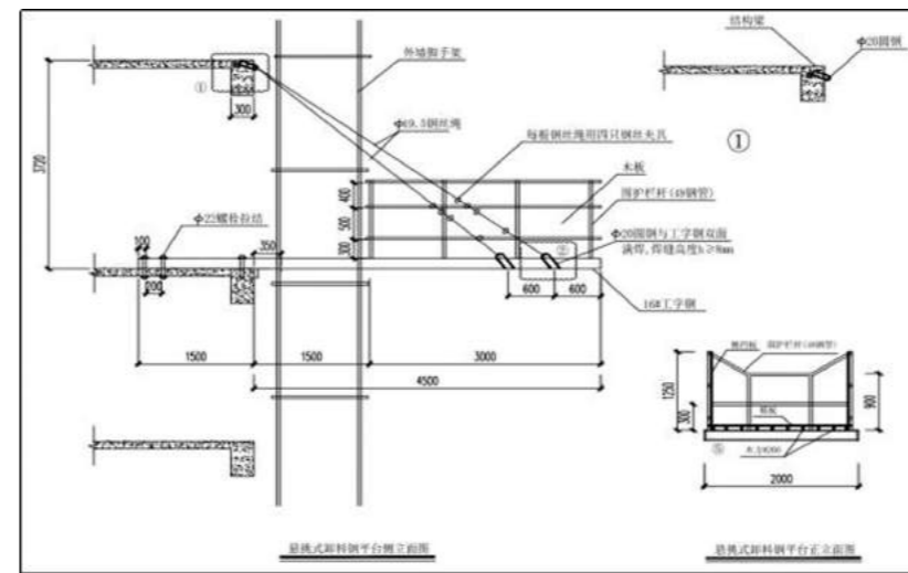
构造简图
